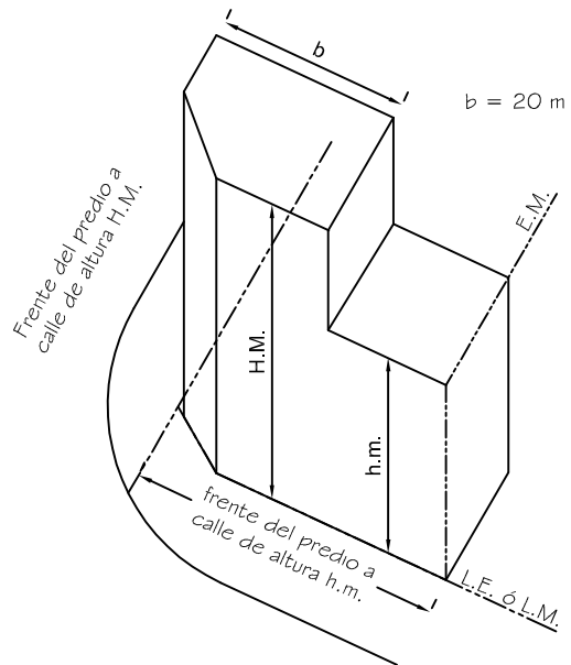
AXONOMETRÍA
